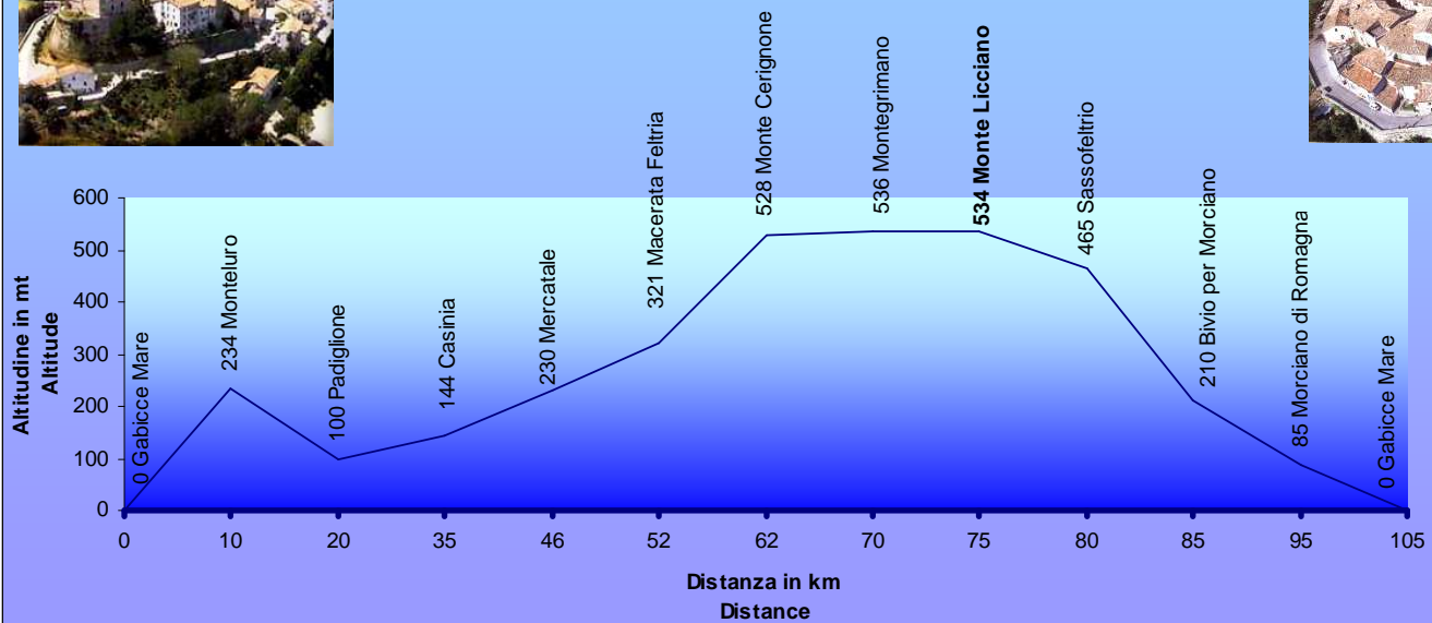
Altimetrie percorso ciclistico "Terme di Montegrimano" Cycling route altimetries Km 105
